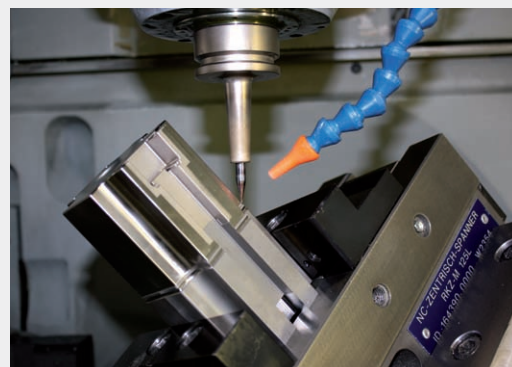
Vollautomatisches Fräsen von komplexen Elektroden
